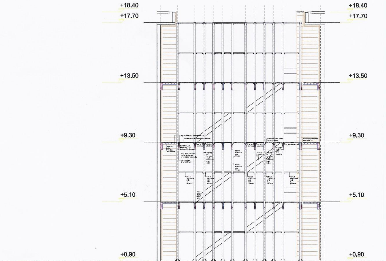
kesit bb ö:1
